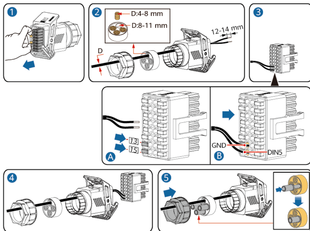
Rysunek 5-23 Podłączanie przewodu
